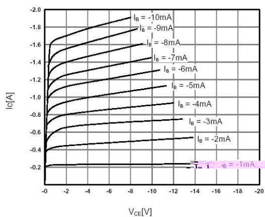
I_C - V_{CE}
