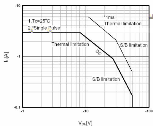
I_C - V_{CE}
