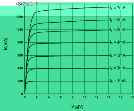
I_C - V_{CE}
